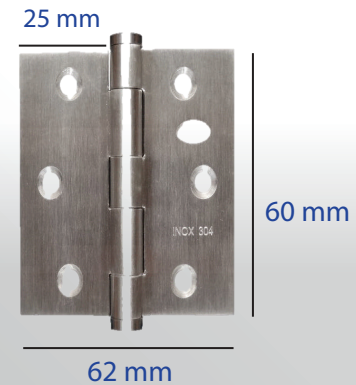
Descripción: BIS.AT.INOX.FIJA Código: 87562
