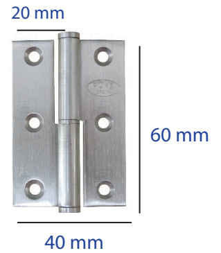
Descripción: BIS.AT.INOX.DESM. Código: 8196040D/I
