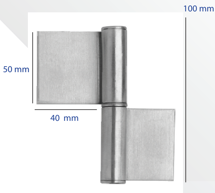
Descripción: BIS. PERNIO. INOX Código: 8180261D/ 8180261I
